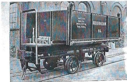
Kippwagen mit eisernem Kastru Spar 1000 mm, Inhalt 5,1 cbm, Leertgewicht 7500 kg, vierkloßige Handspindelbremse Geliefert an die Allgemeine Deutsche Kleinbahn-Gesellschaft A.-G. Berlin für die Bieberthalbahn Gießen
